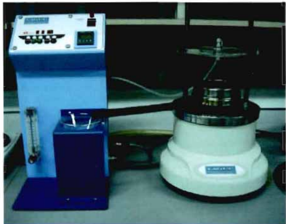
Ensayo para la determinación de la medida de abertura característica EN ISO 12956. Laboratorio de Ensayos de Geosintéticos de la Universidad de Cantabria (LAGUC).
