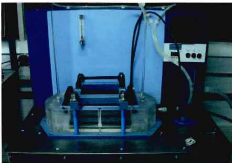
Ensayo para la determinación de la capacidad de flujo en su plano UNE - EN ISO 12958. Laboratorio de Ensayos de Geosintéticos de la Universidad de Cantabria (LAGUC).
